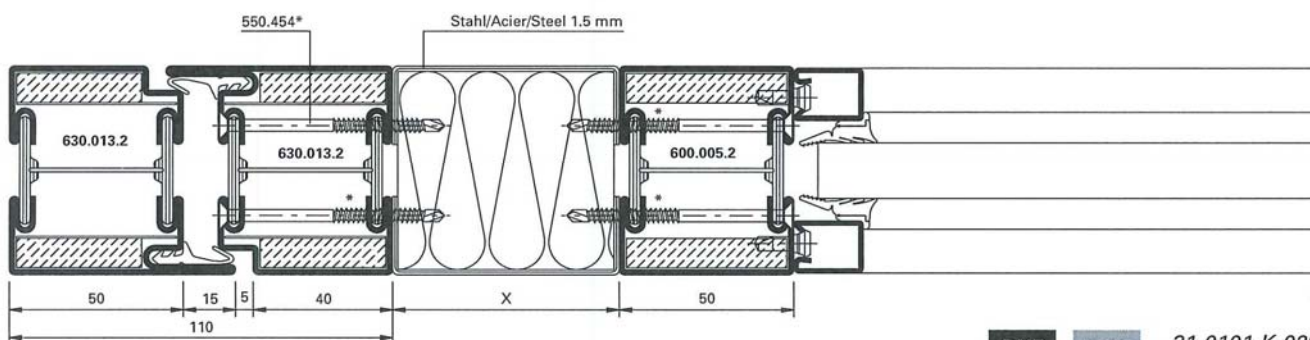
Türflügel-Aufdoppelung
