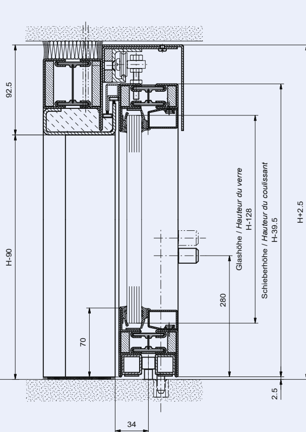
Vertikalschnitt Schieber Coupe verticale coulissants
