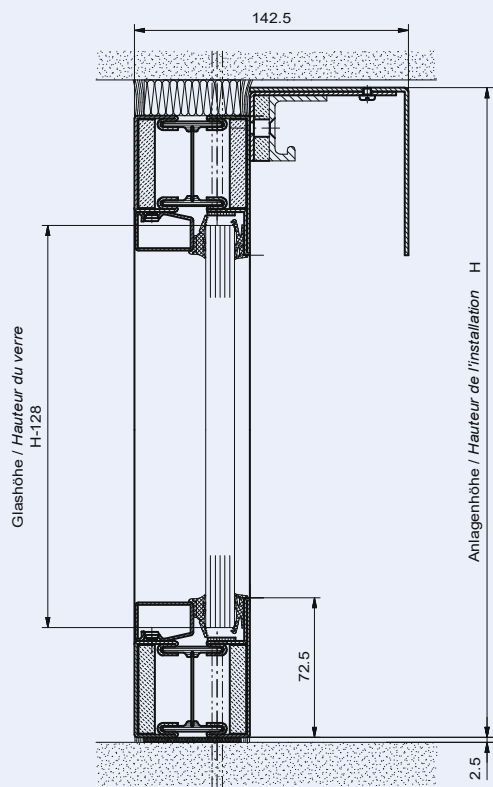
Vertikalschnitt fester Teil Coupe verticale partie fixe
