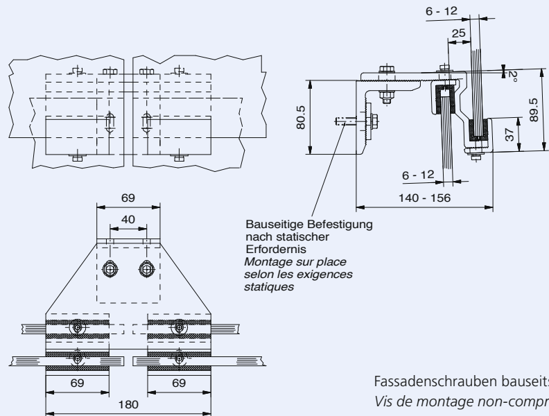
Fassadenschrauben bauseits Vis de montage non-comprises
